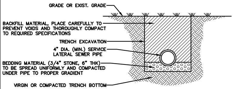
STANDARD LATERAL DETAIL 3'-8' IN DEPTH N.T.S.
