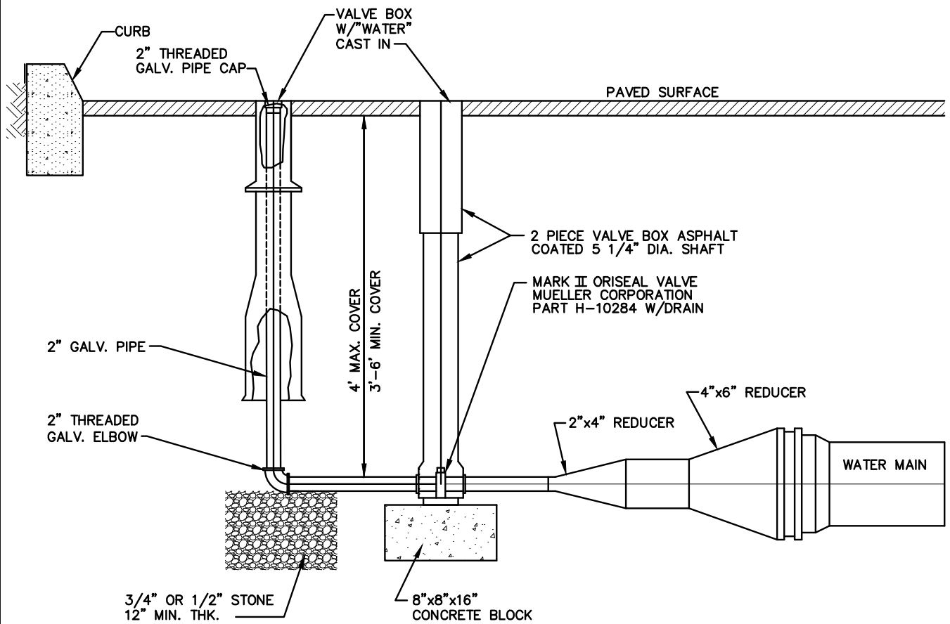
BLOW-OFF DETAIL N.T.S.
